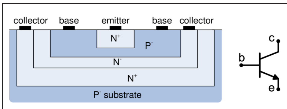
Tasomaisen NPN BJT:n yksinkertaistettu poikkileikkaus
